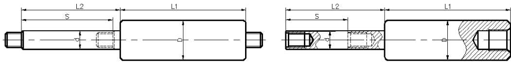
L1-缸筒长度 L2-活塞杆伸出长度 D-缸筒直径 d-活塞杆直径 S-行程
